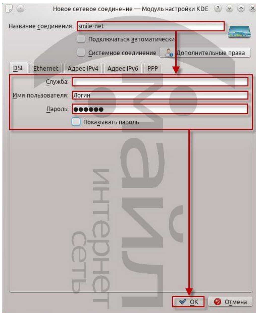
Рисунок 3. Создание PPPoE подключения
